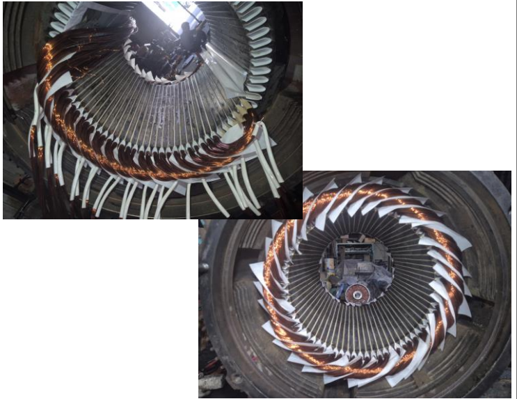
STATOR 권체
