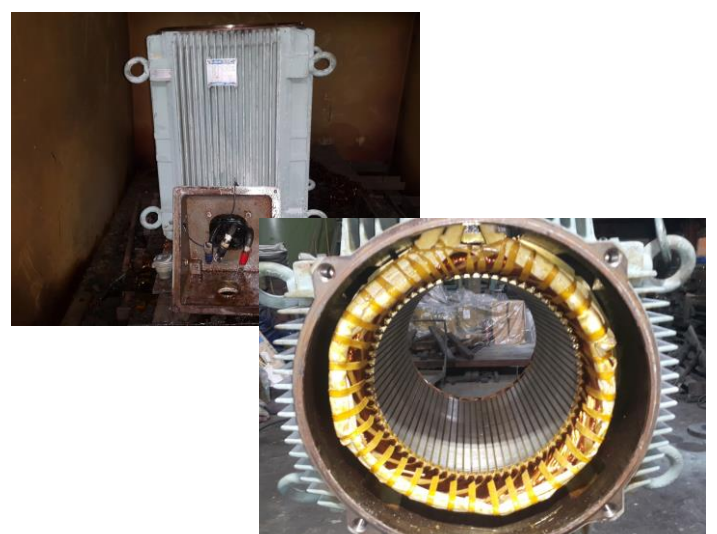
STATOR권체
