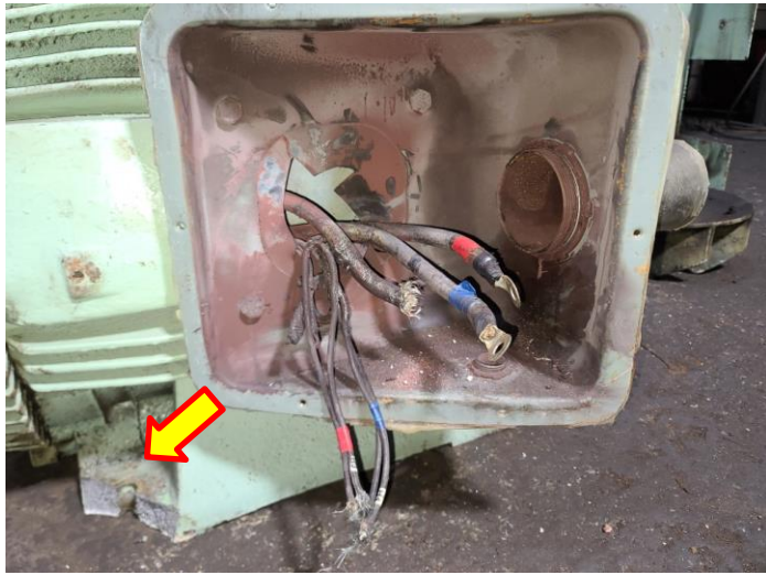
입고검사
