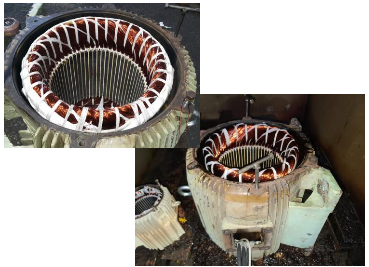
STATOR 권체
