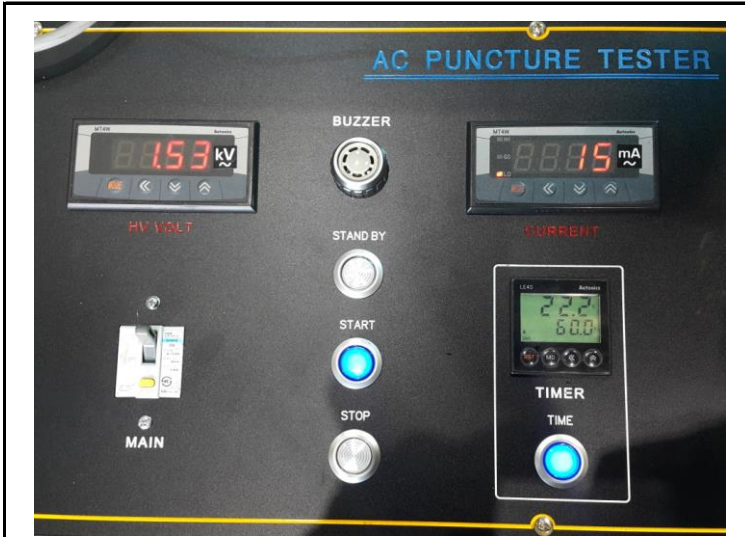
출고검사
