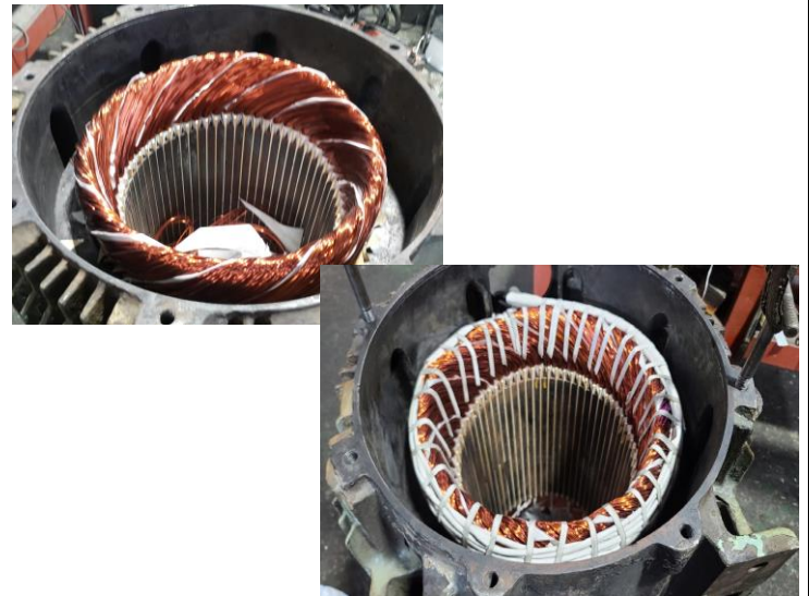
STATOR 권체
