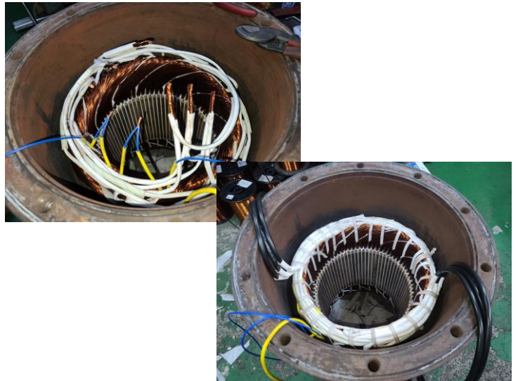
STATOR권체
