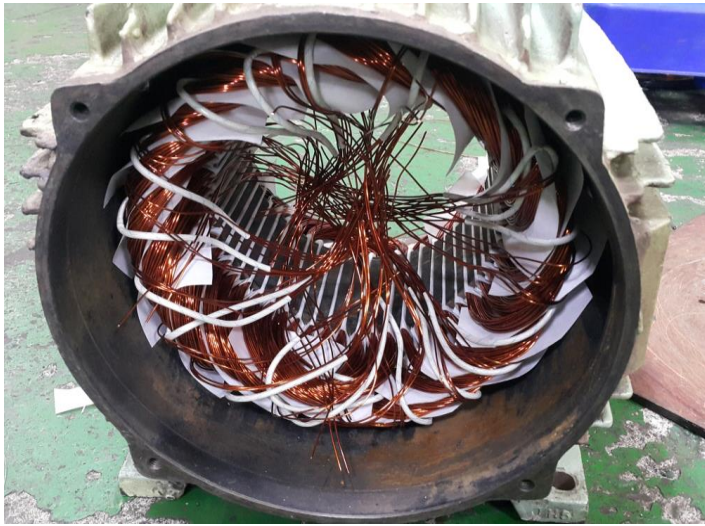
STATOR권체
