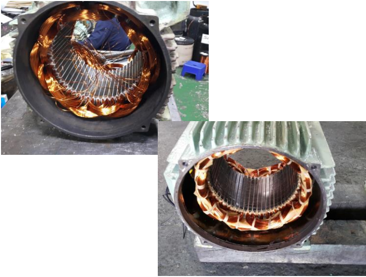
STATOR권체
