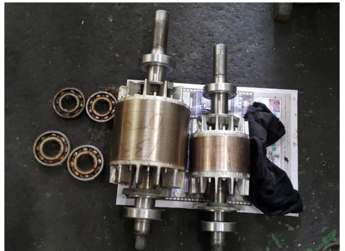
ROTOR
