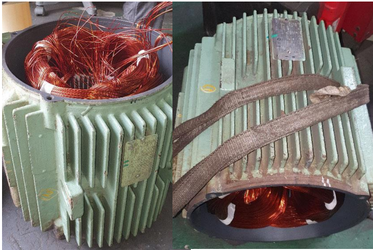
STATOR권체
