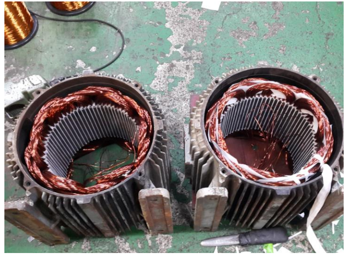
STATOR권체
