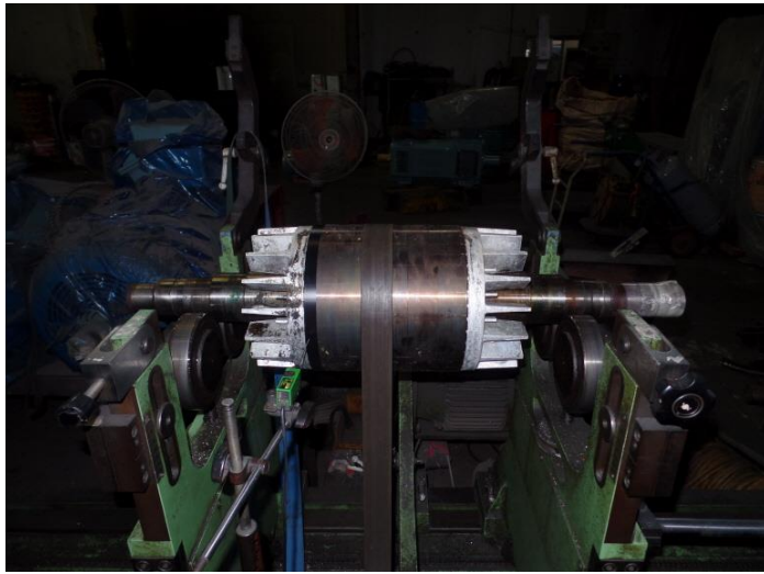
ROTOR
